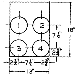
4-5 CONDUITS 5 1/2 O.D.
