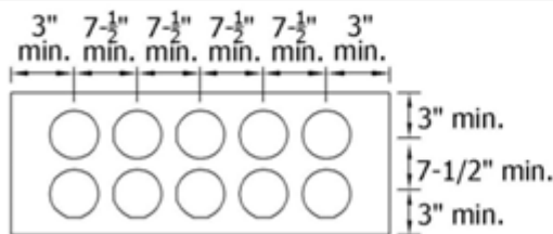
Conduit placement for maximum number of conduits
