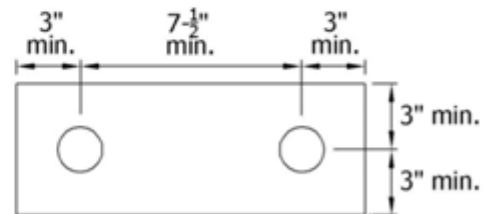
Conduit placement
